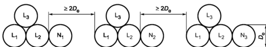
Рисунок Н.52.5 - Специальная конфигурация для девяти параллельных одножильных кабелей один выше другого (см. 523.7)
